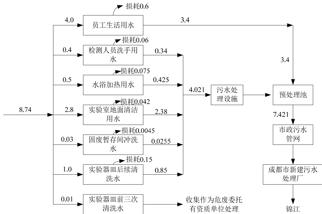
图 2-1 项目水平衡图 (消耗单位: m³/d)
