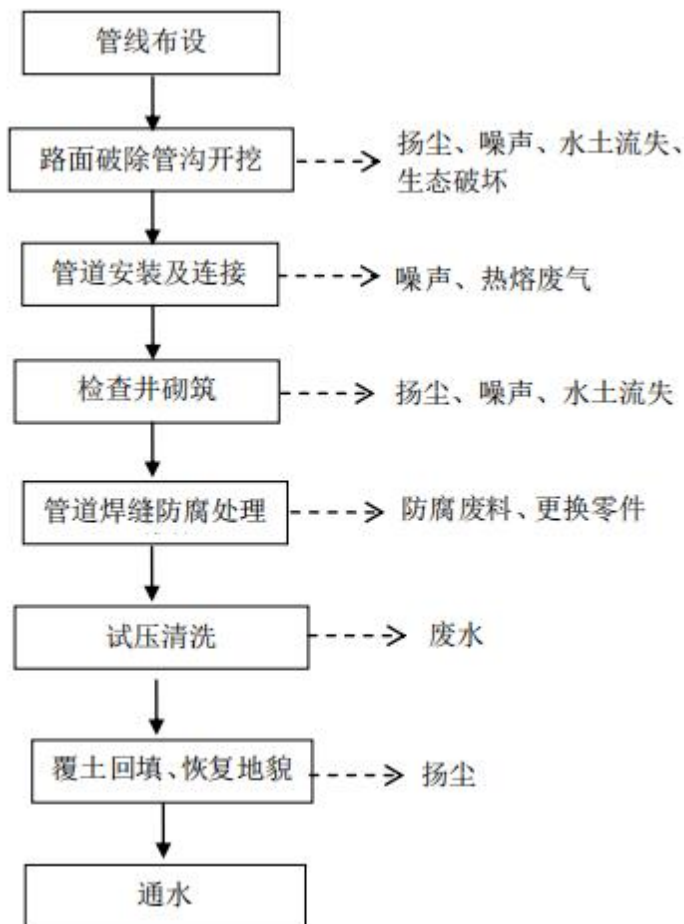
图 4-1 管网施工流程及产污环节图
